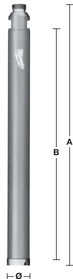
WCHP-SB Ø 52–152 mm
