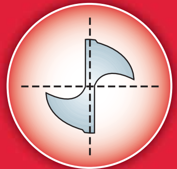
Tværsnit af en traditionel borkrop
