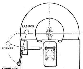
Tre-punkts bremse
