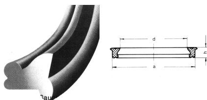
Storz sugepakning
